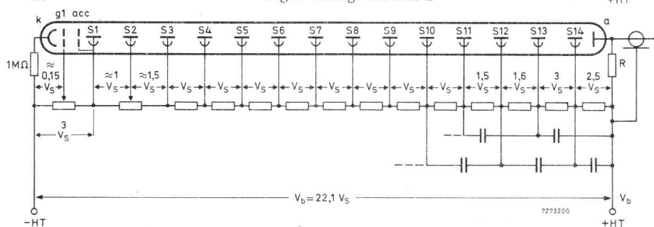
Fig. 3 Voltage divider B'
